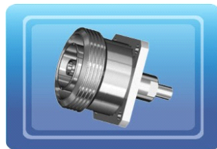
产品型号: L29-50KF33 相配电缆: SFT-50-3 RG141
