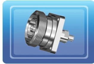
产品型号: 7/16-50KF4.5 相配电缆: SFF-50-3 RG402
